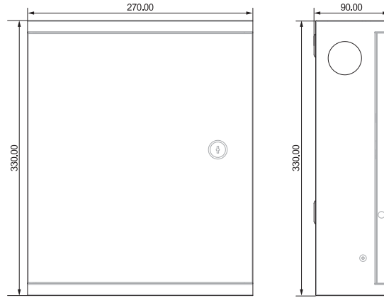
图1-1 外观尺寸
