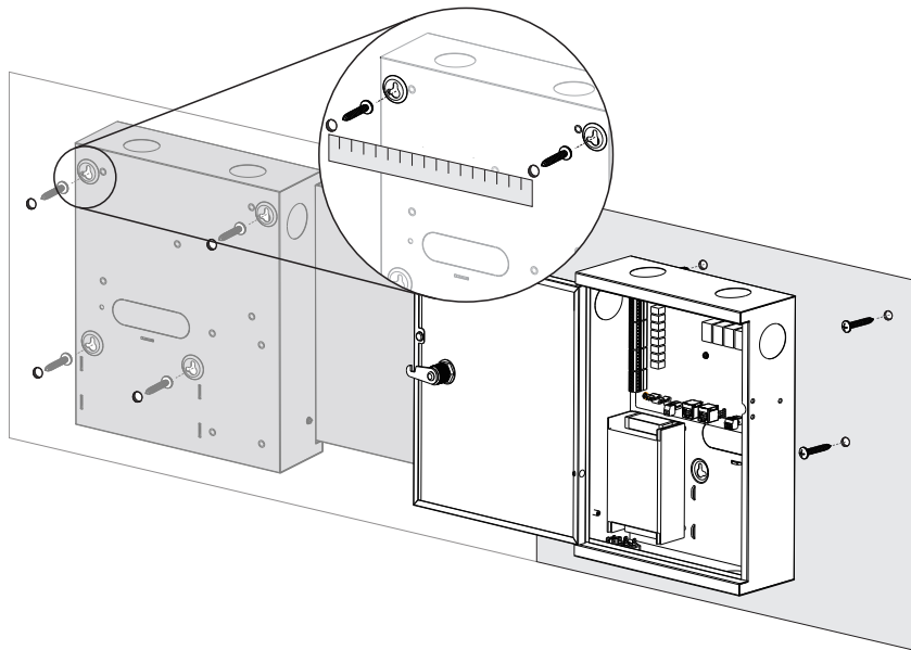
图3-3 安装示意图
